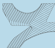
Scan-Path berechnen
